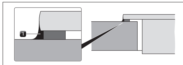
Obr. 5.18 silikónová tesniaca hmota pri montáži na povrch
