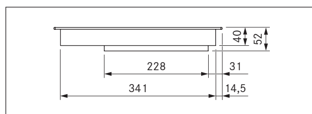
Obr. 3.3 Rozmery varnej dosky PKFI11, pohľad spredu
