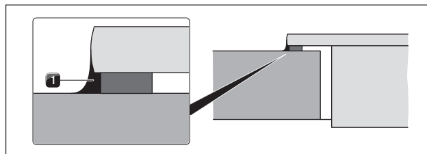
Obr. 5.17 silikónová tesniaca hmota pri montáži na povrch
