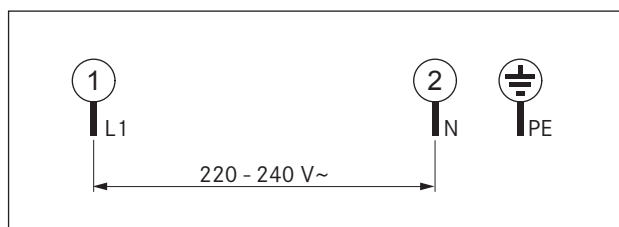
Obr. 5.20 Schéma zapojenia 1-fázové
