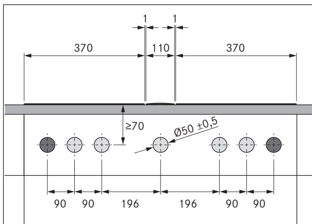
Obr. 5.13 Otvory dosky ovládacieho panela pri 2 varných doskách a 1 odťahu
