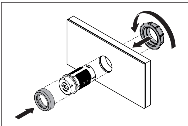
Obr. 5.12 Montáž ovládacieho kolieska
