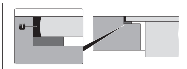
Obr. 5.18 silikónová tesniaca hmota pri zapustenej montáži
