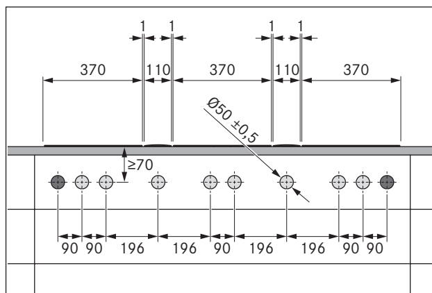
Obr. 5.14 Otvory dosky ovládacieho panela pri 3 varných doskách a 2 odťahoch
