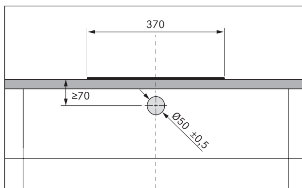
Obr. 5.11 Vŕtacia šablóna
