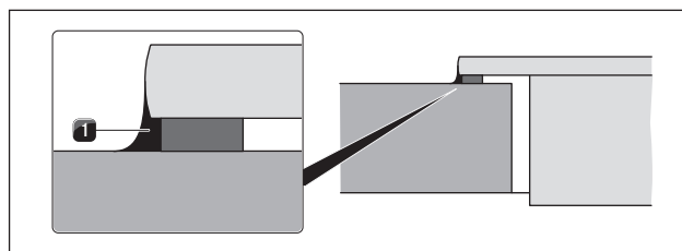
Obr. 5.19 silikónová tesniaca hmota pri montáži na povrch
