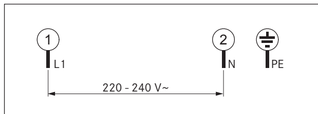
Obr. 5.22 Schéma zapojenia 1-fázové
