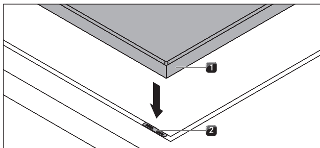
Obr. 5.16 Varná doska a podložky na nastavenie výšky
